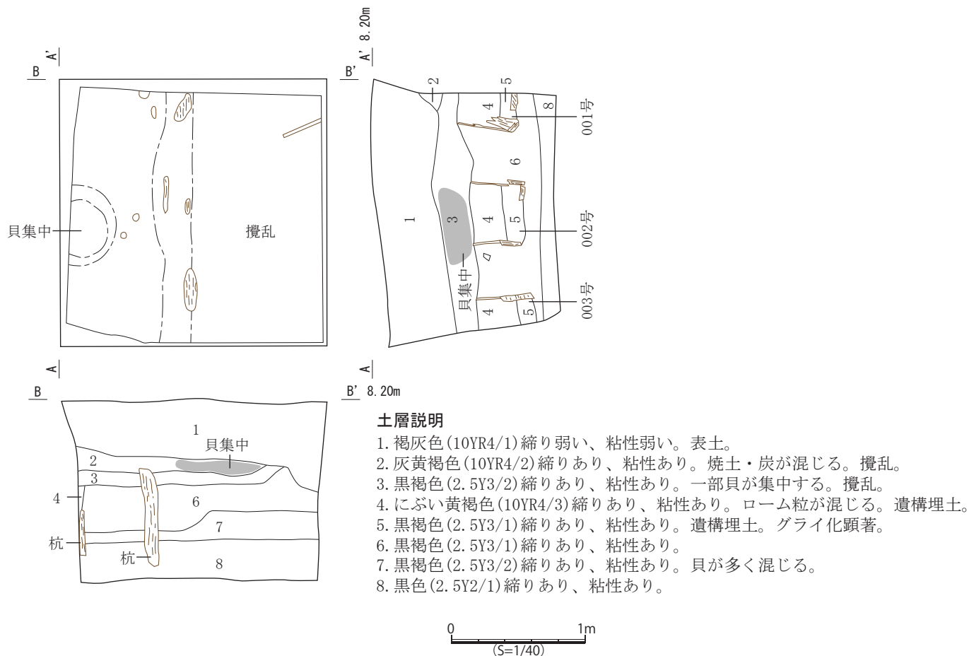
第3図 試掘坑平面図・断面図 (S=1/40)
