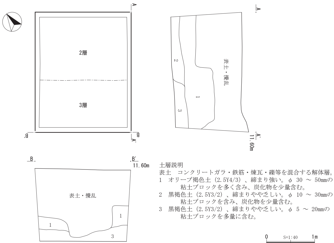
第3図 試掘坑平面図・断面図 (S=1/40)
