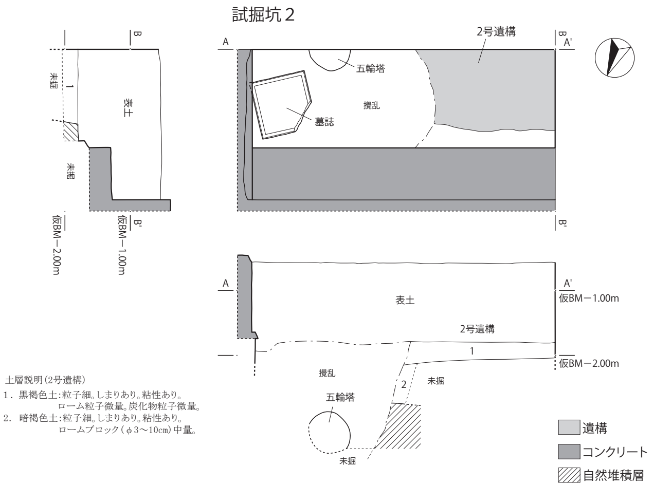
第4図 試掘坑1・2 平面図・断面図 (S=1/60)
