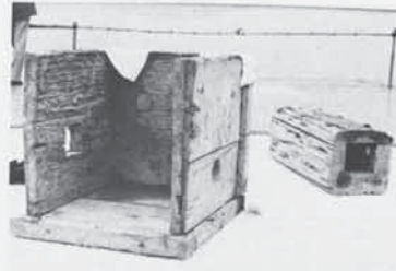
（神田上水の木管と留柄）
