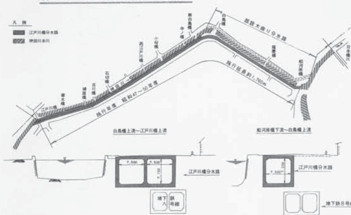
神田川江戸川橋分水路平面図
