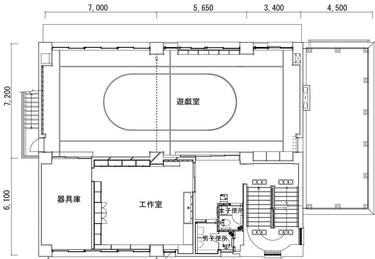
3階平面図 S=1/150
