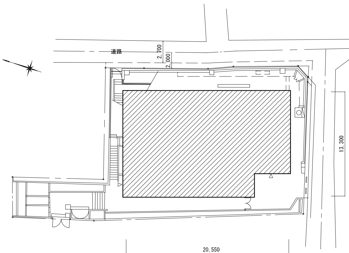
配置図 S=1/300
