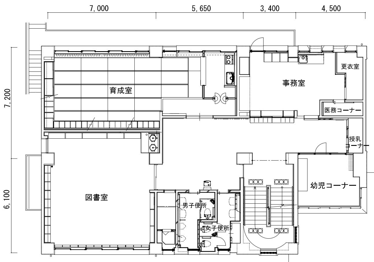
2階平面図 S=1/150
