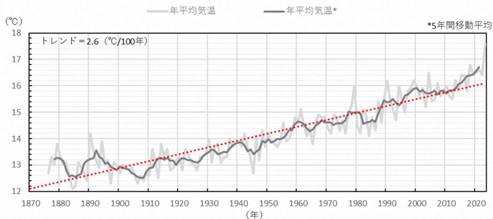
出典 関東甲信地方のこれまでの気候の変化（観測成果）（東京管区气象台）より作成 図 3 東京都（東京気象観測所：千代田区）の年平均気温の経年変化
