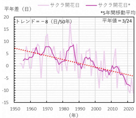
図 5 東京管区気象台のサクラ開花日・カエデ紅葉日の経年変化
